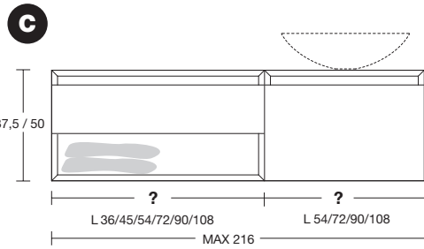
VERSIONE DX - Right version - Version rechts Version droite - Versión derecha - Прав. вариант
