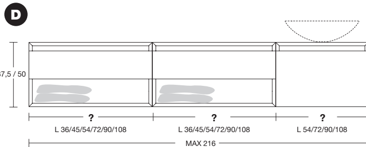
VERSIONE DX - Right version - Version rechts Version droite - Versión derecha - Прав. вариант
