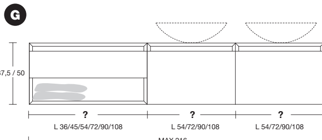
VERSIONE DX - Right version - Version rechts Version droite - Versión derecha - Прав. вариант
